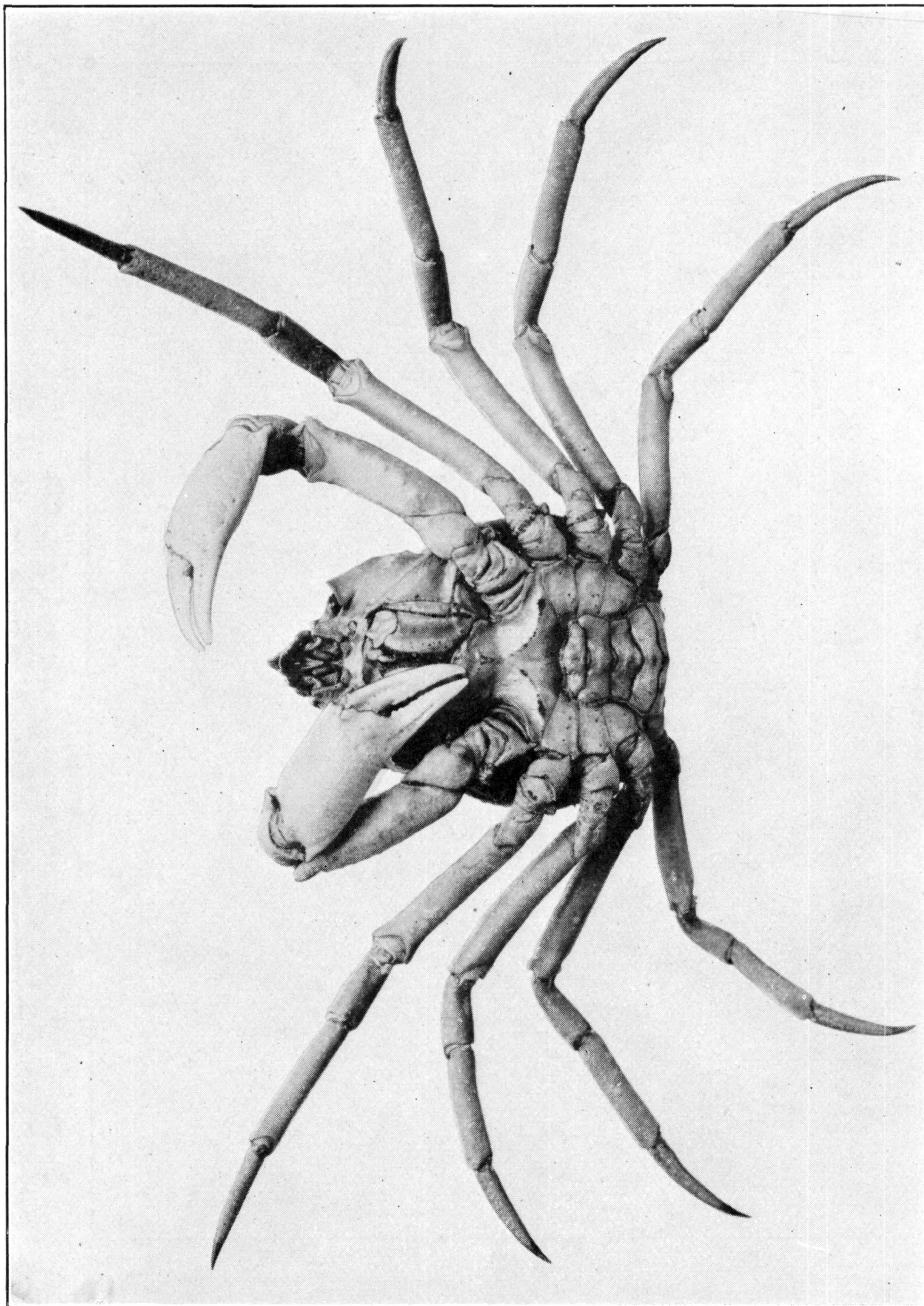
HYAS ARANEUS. (PAGE 253)
