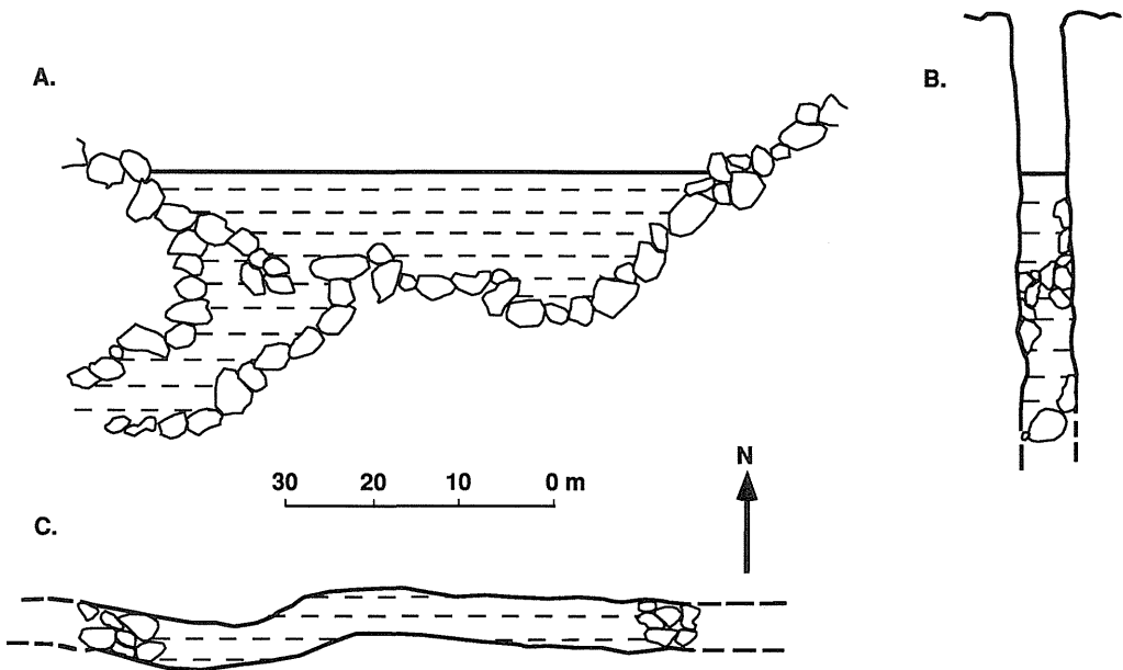
Fig. 3. Profile (A), section (B), and plan (C) maps of Grieta de Caleta la Torta, Isla Santa Cruz, Islas Galápagos. (Drawn by Thomas M. Iliffe.)
