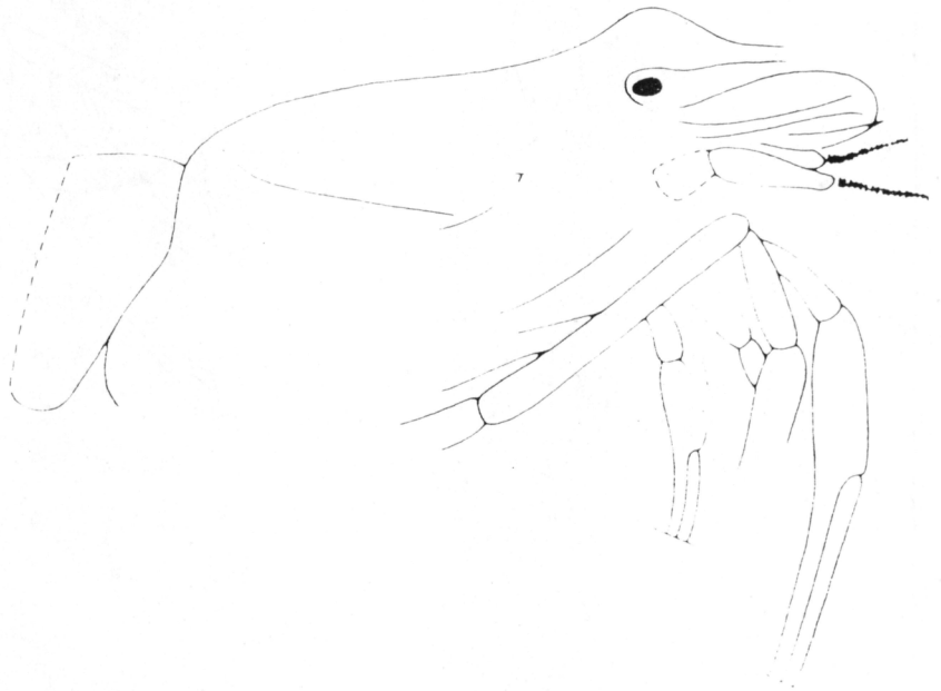
Fig. 13. Baica strachoni n. sp. n. cat. MSNM 111203: photo. and reconstruction (x 45).
