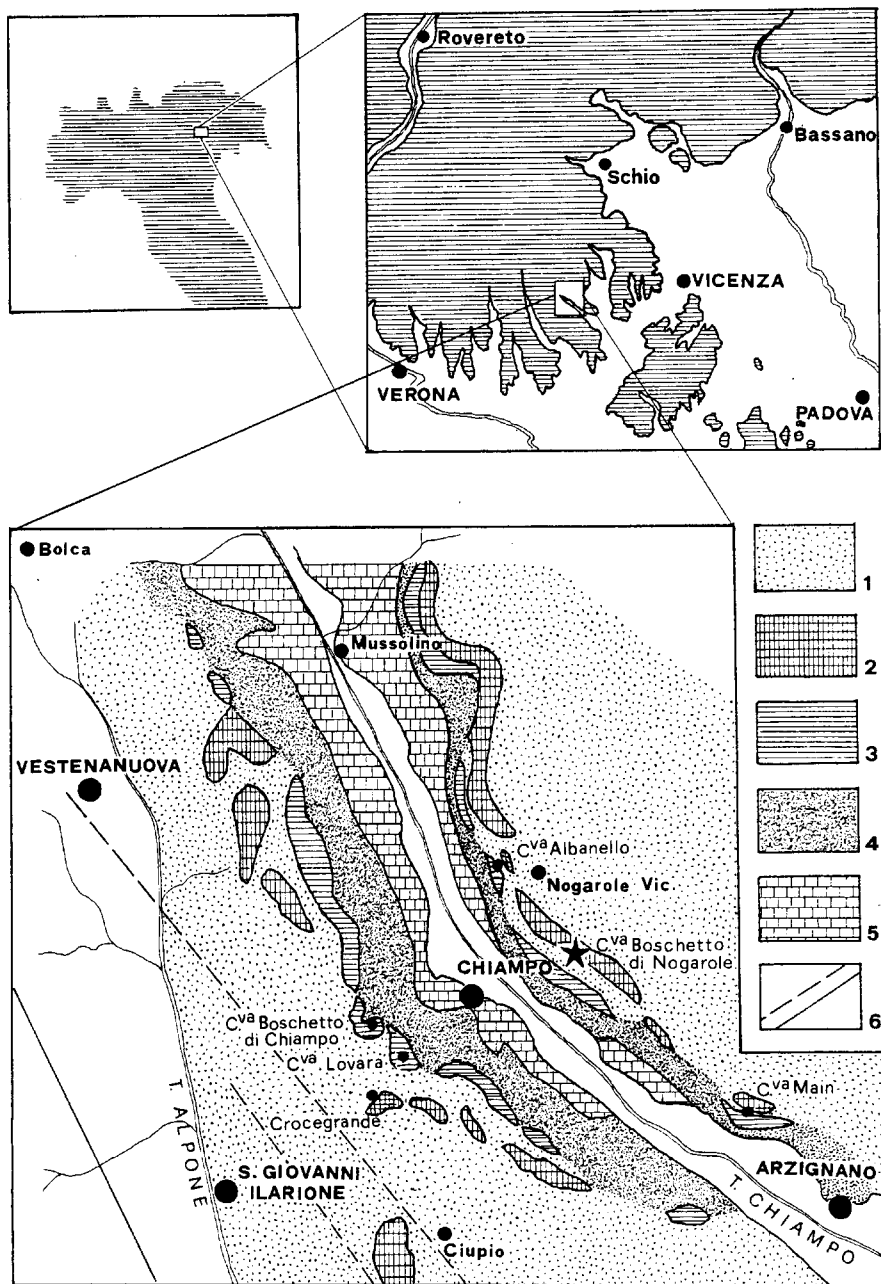
Fig. 1 - Posizione geografica e schizzo geologico della parte media della Valle Chiampo (Vicenza) (da DE ZANCHE, 1965 - modificato). 1) Vulcaniti superiori; 2) Calcari nodulari del Luteziano medio e superiore; 3) Calcari massicci del Cuisiano e del Luteziano inferiore; 4) Vulcaniti inferiori; 5) Scaglia e Biancone; 6) Faglie accertate e presunte.
